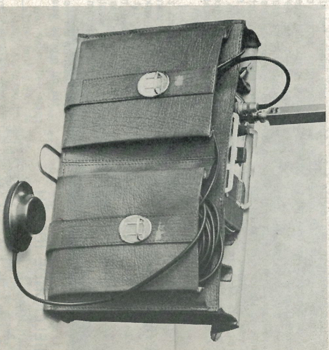
De marifoon in tas, zoals de loods hem meeneemt. Door de uitklapbare voetbeugel kan het geheel rechtop staan.
