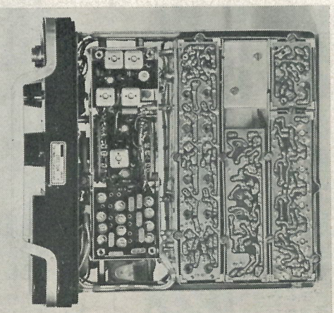
Het inwendige van de HTC 3307. Het apparaat is opgebouwd uit gedrukte schakelingen, die aan twee zijden van een frame zijn aangebracht.
